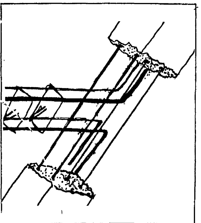
Anclaje de columneta nueva en viga existente
