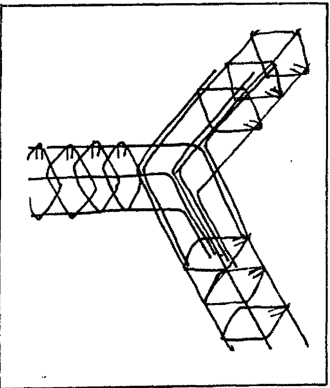
Unión de columneta con vigas de amarre en esquina
